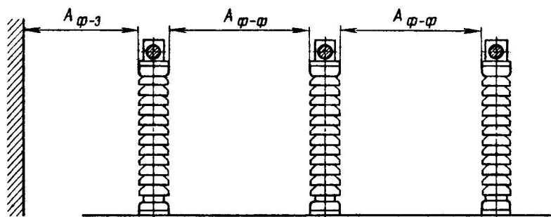
Рис. 4.2.1. Наименьшие расстояния в свету при жестких шинах между токоведущими и заземленными частями ( A_{ф-з} ) и между токоведущими частями разных фаз ( A_{ф-ф} )
